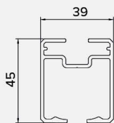
Guides latéraux Schiebemarkise
