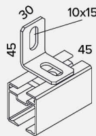
Fixation sur support Befestigung zwischen zwei Wänden
