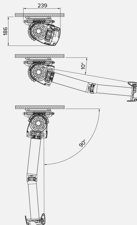
Fixation au plafond . Deckenbefestigung
