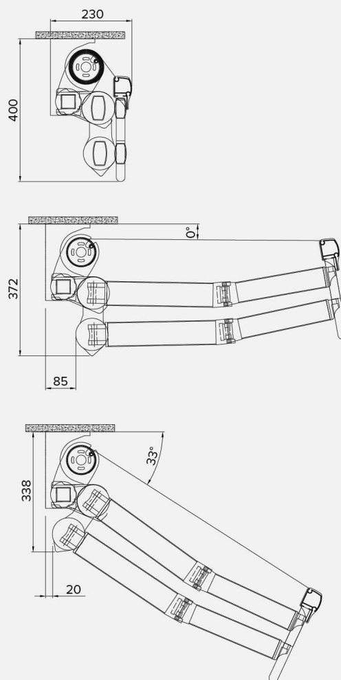
Fixation au plafond . Deckenbefestigung
