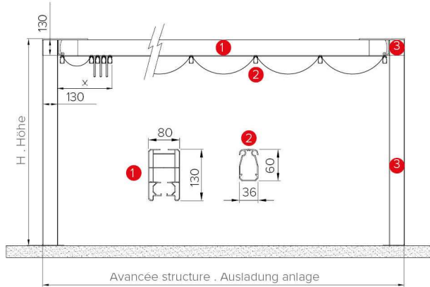
Vue latérale . Seitenansicht
