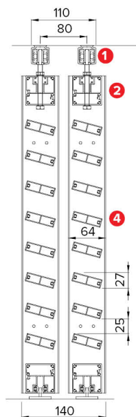
Doghe in alluminio inclinazione 15° Aluminium slats 15° inclination
