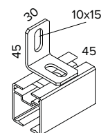
Attacco spallina Fixation latérale
