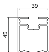
Guide Laterali Coulisses latérales
